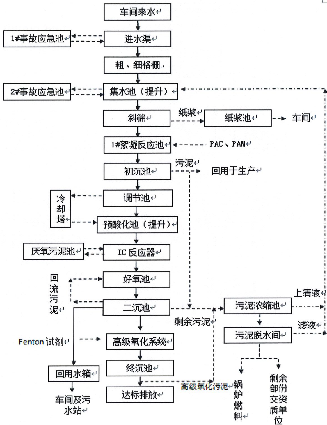
东莞金洲纸业有限公司一厂区废水处理流程图
