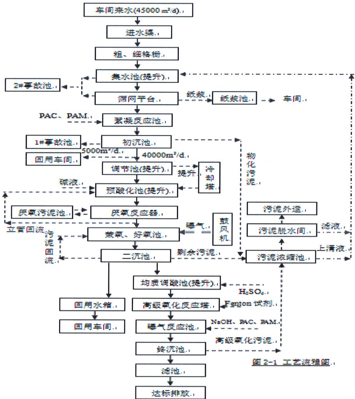
东莞金洲纸业有限公司二厂区废水处理流程图
