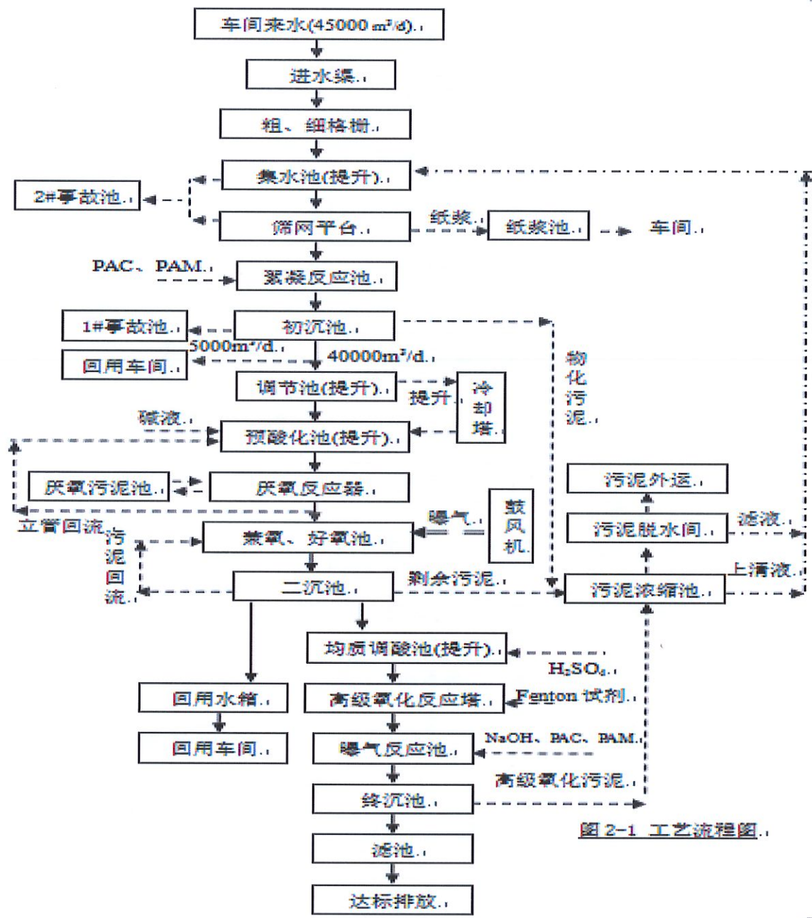
东莞金洲纸业二区废水处理流程图
