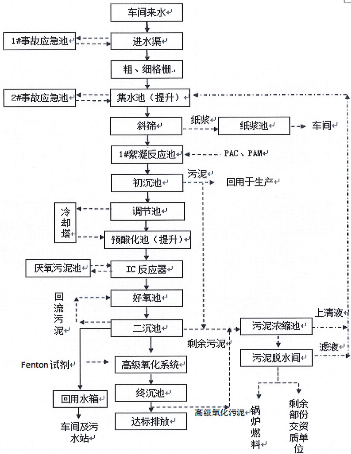
东莞金洲纸业有限公司一区废水处理流程图
