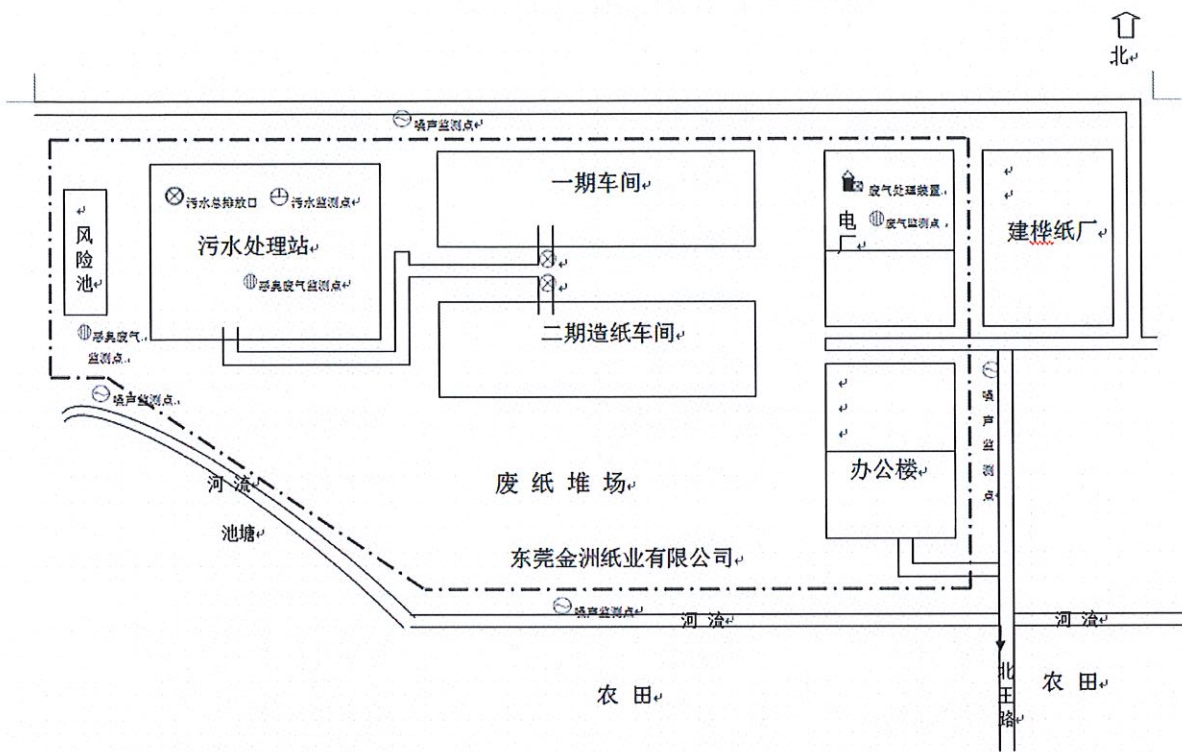
东莞金洲纸业有限公司一区平面布置及监测点位分布图
